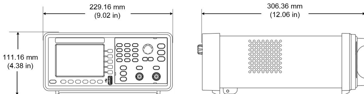
Рис. 1. Размеры прибора
